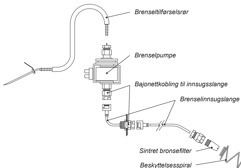
Brenselssystemets bestanddeler
