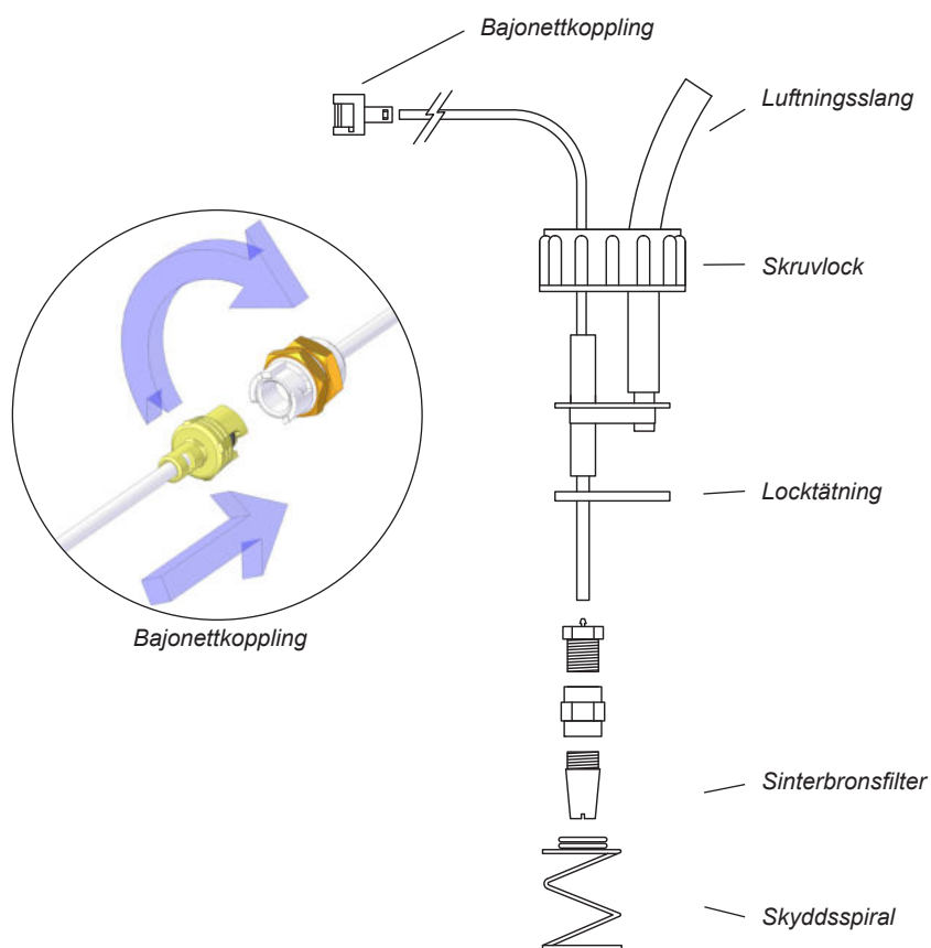
Lockförsedda genomföringar
