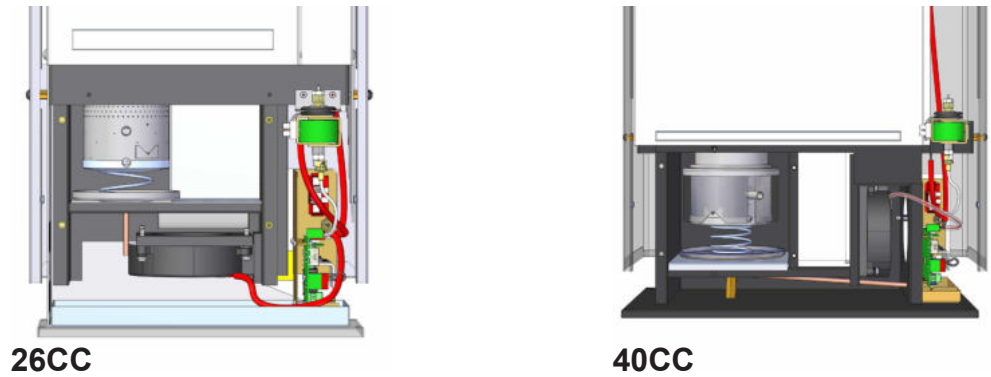
Poltinkotelo avattuna
