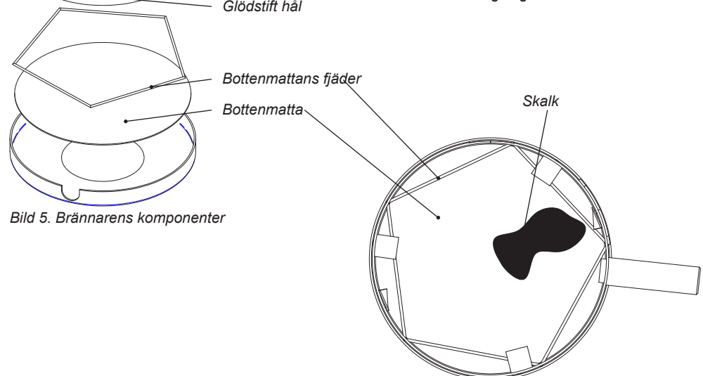
Bild 7. Brännarcylinder
