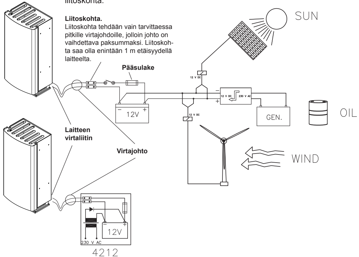
Sähköjärjestelmän periaatekuva.
