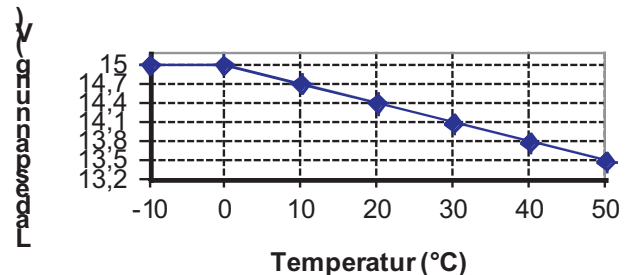
Temperaturabhängigkeit der Gasungsspannung einer 12V-Blei-Gel-Batterie
