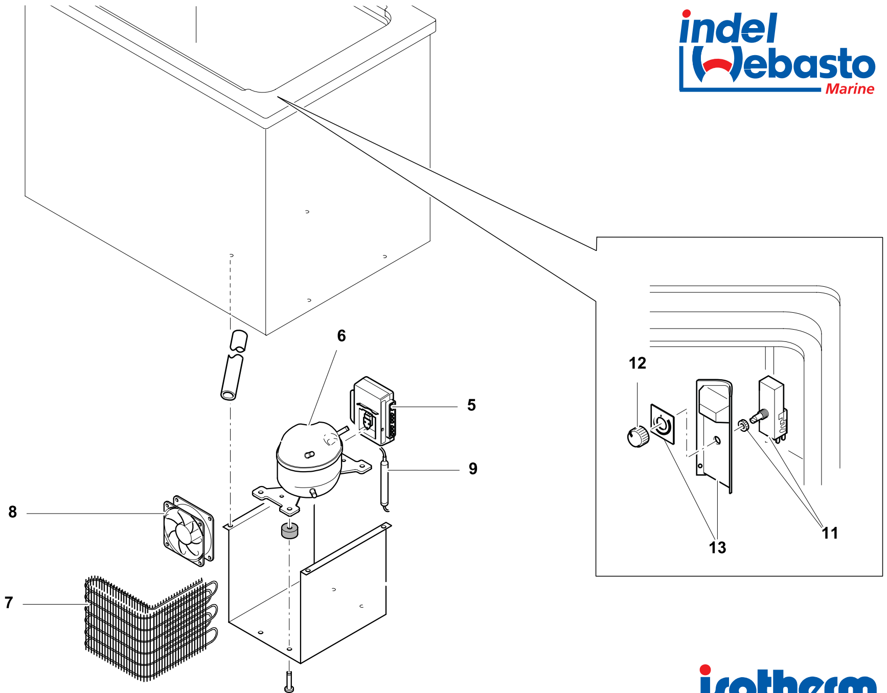
BI 41 - COOLING UNIT
